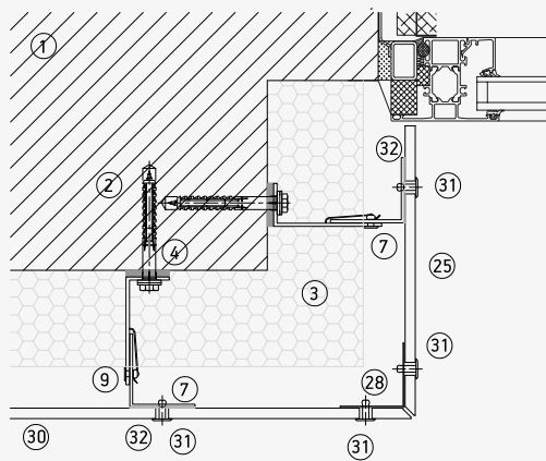
Jamba Dekton
