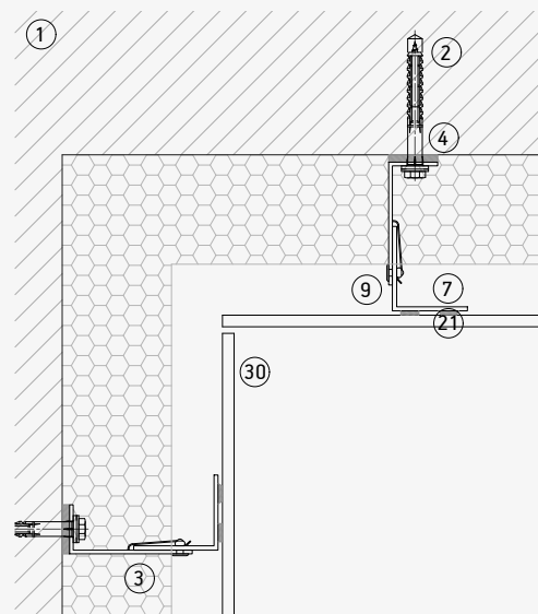
Esquina interior
