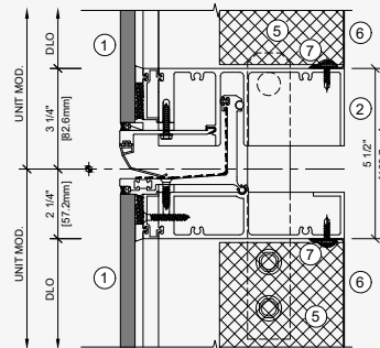
Junta Horizontal
