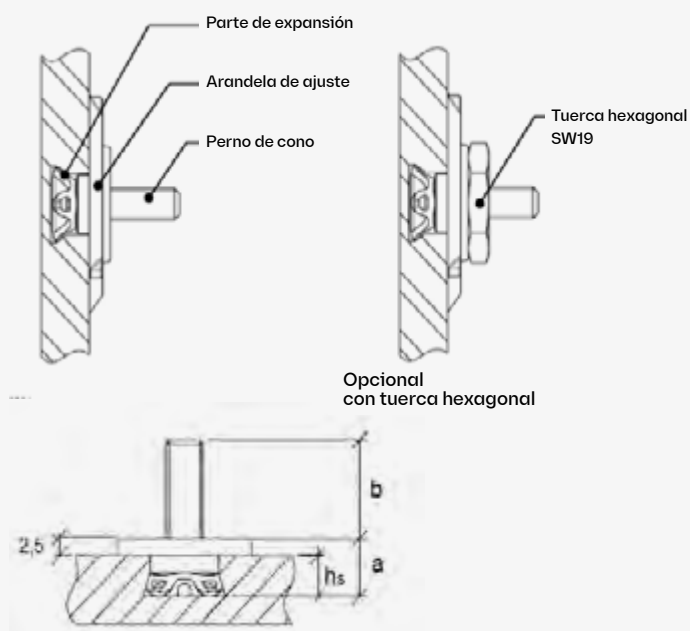
FISCHER FZP II Anclaje destalonado (DKT1.2)
