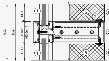
Junta Horizontal
