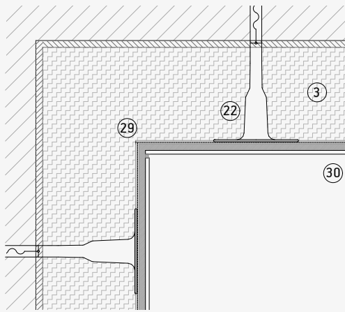
Esquina interior
