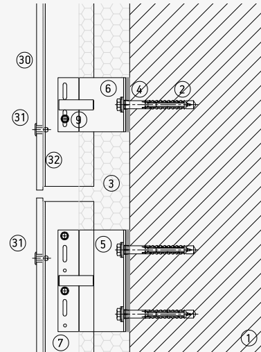
Junta horizontal dilatación
