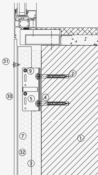
Arranque ventana
